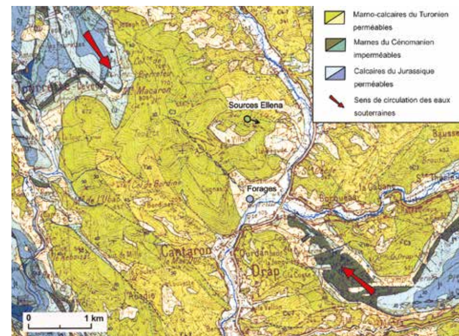
Extrait de la carte géologique au 1/50 000 de Menton - Nice (éditions du BRGM)
