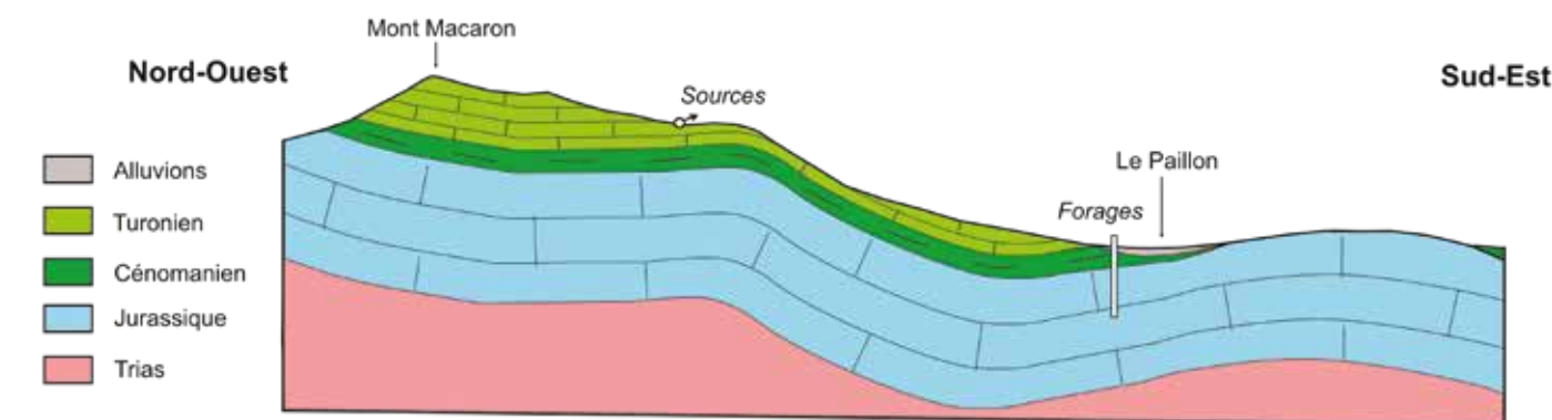
Coupe géologique simplifiée avec la localisation des sources et des forages de Cantaron
